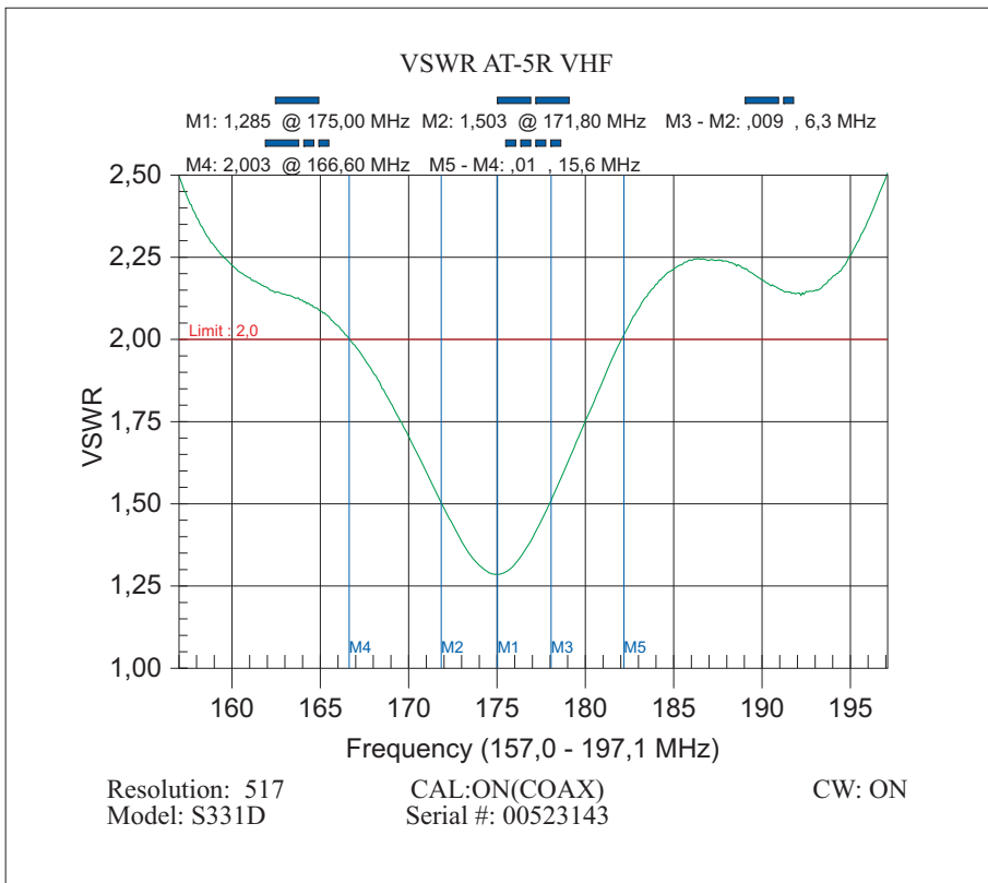
Типовое КСВ для F(C)=175 МГц
