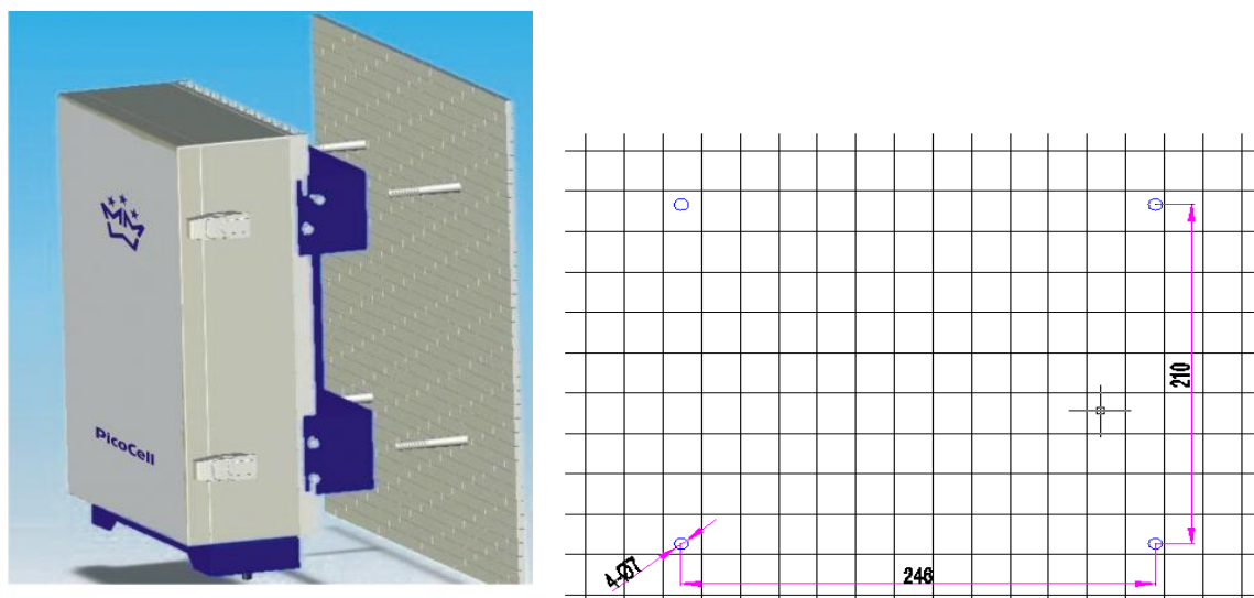
Схема установки.
