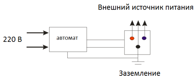
Схема подключения источника питания.
