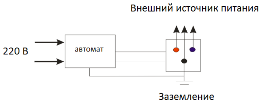
Схема подключения источника питания.
